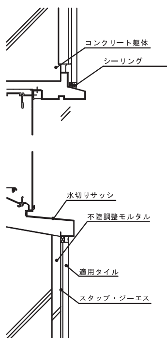
【出隅部】
