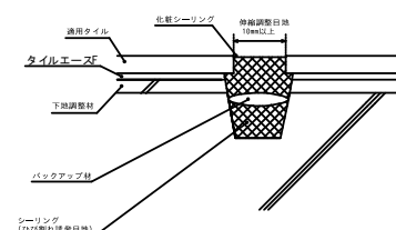
伸縮調整目地の設置例
