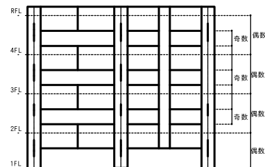
外装タイル垂直方向の割付け
