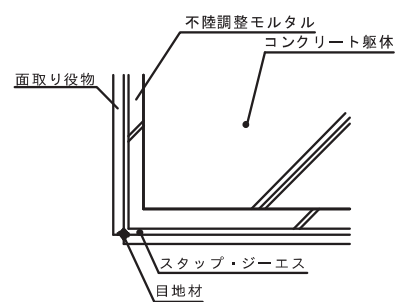
【開口部水平断面】
