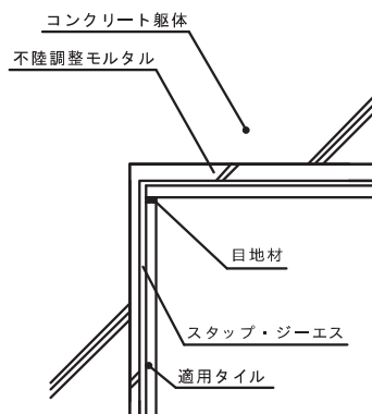
【入隅部】
