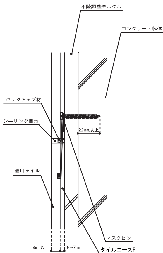
【鉛直断面】
