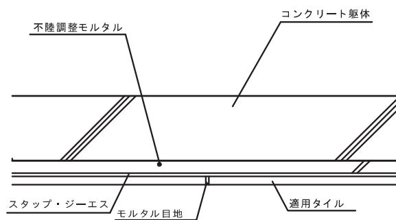
【入隅部】
