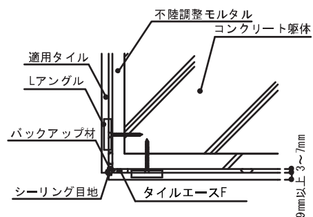
【出隅部】
