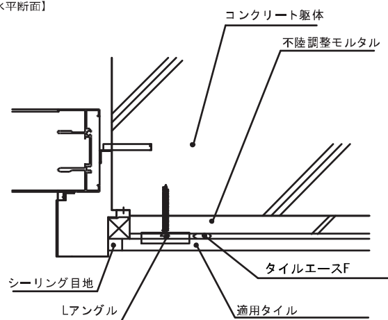
【開口部水平断面】
