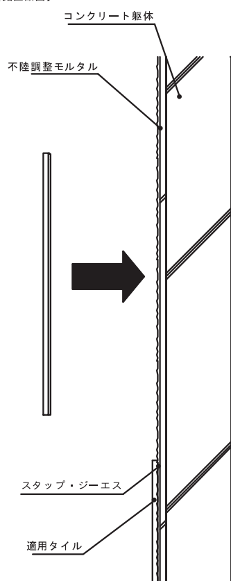
【鉛直断面】
