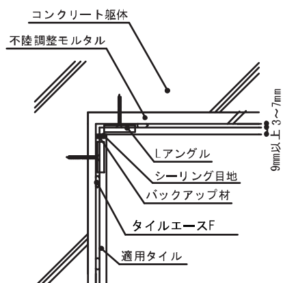
【入隅部】
