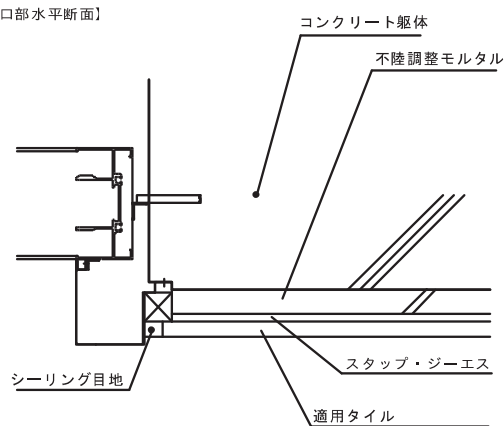
【開口部水平断面】
