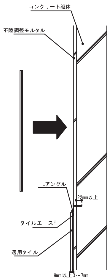
【鉛直断面】
